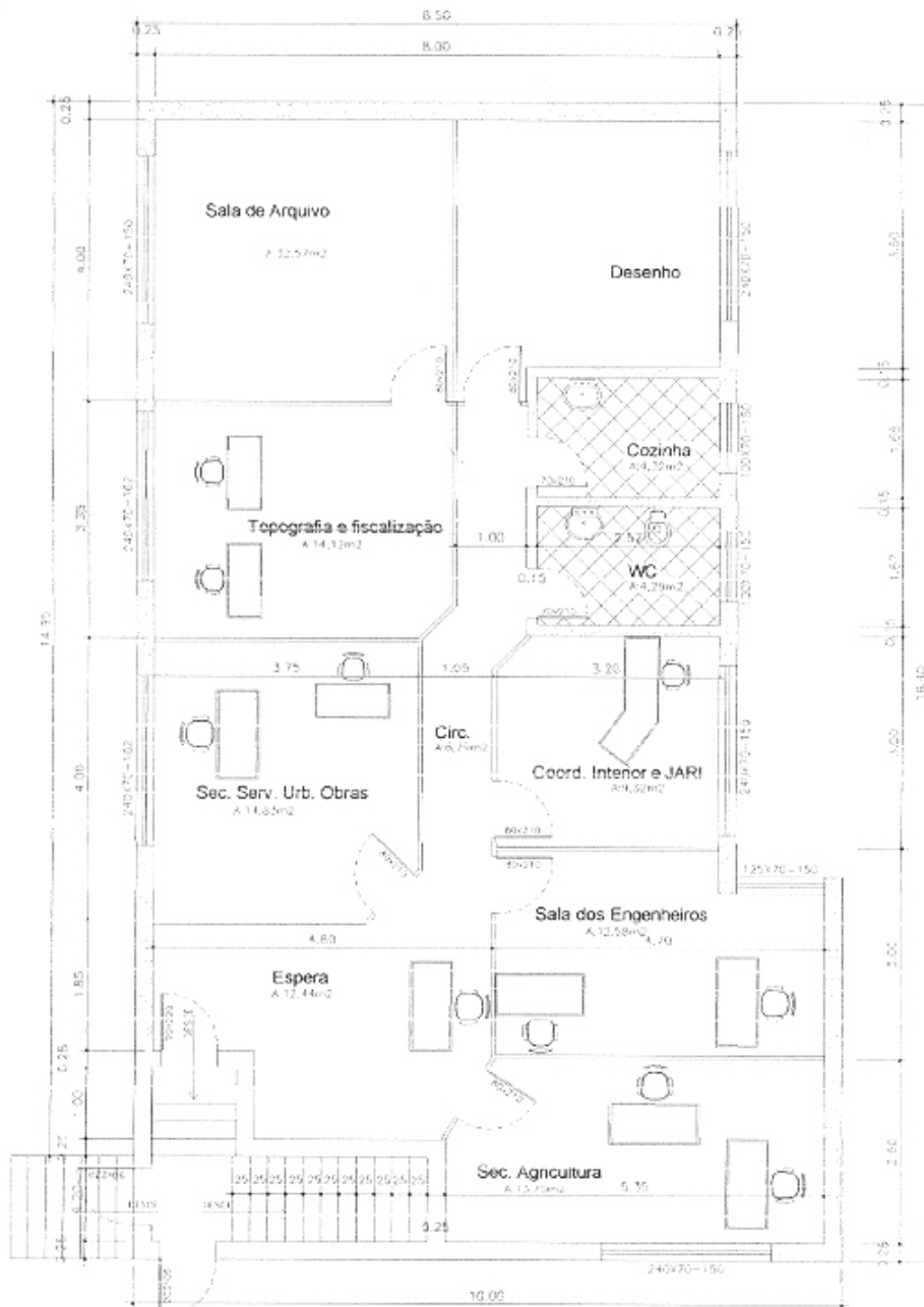
Planta Baixa- PAVTO SUPERIOR ÁREA: .....147,57m 2
