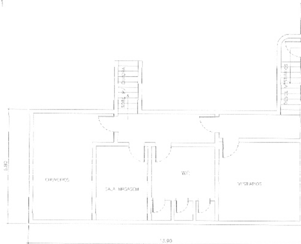
PLANTA BAIXA-VESTIÁRIOS 2X
