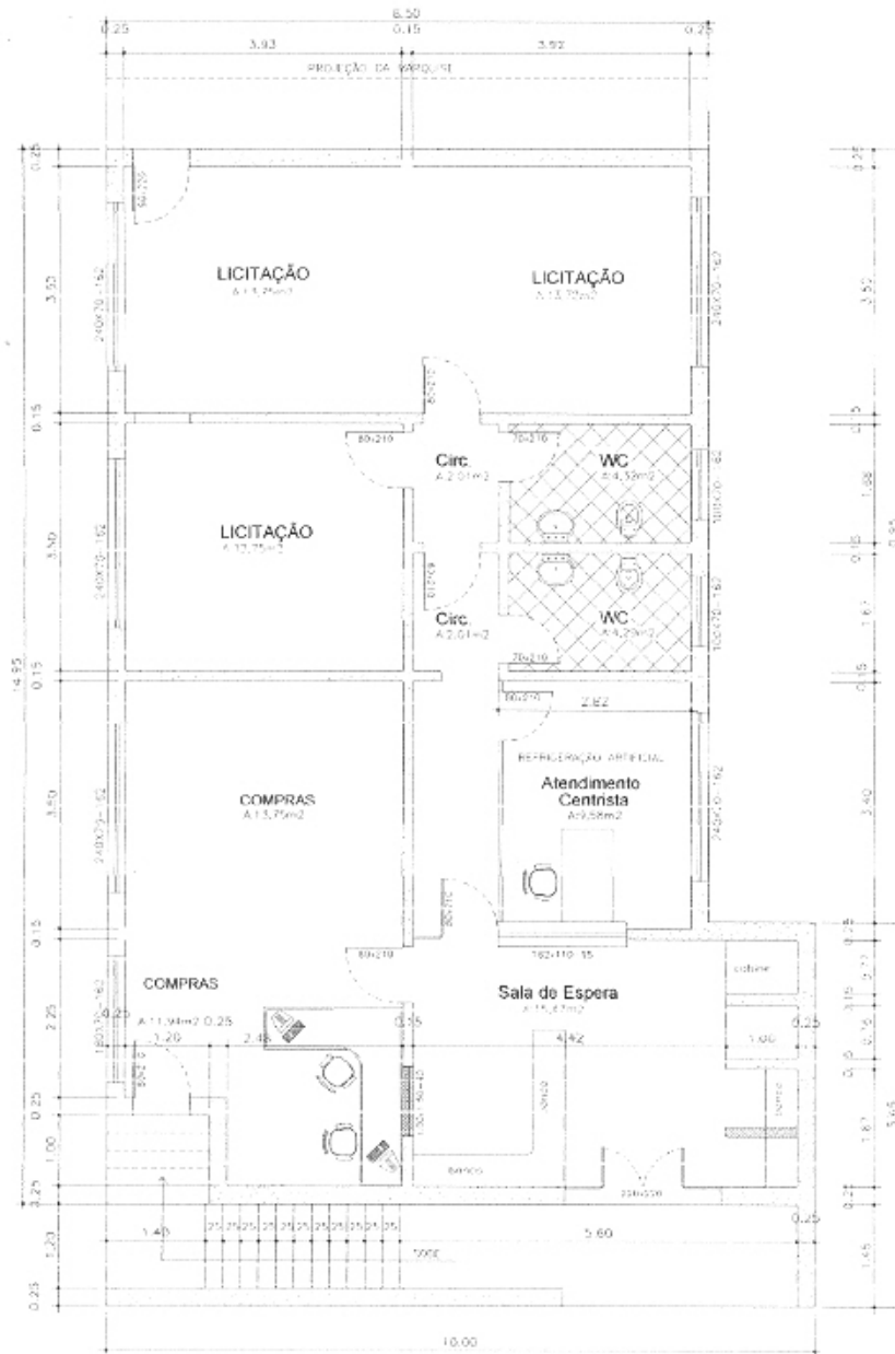
Planta Baixa- PAVTO INFERIOR ÁREA: .....147,57m 2
